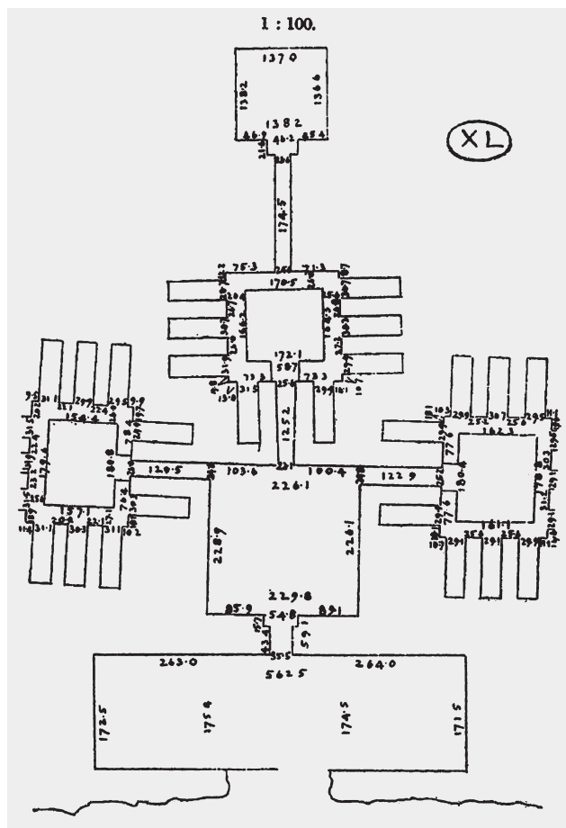
Рис. 5. План пещеры Руммание У.-М.-Ф. Петри. 1890 г.
